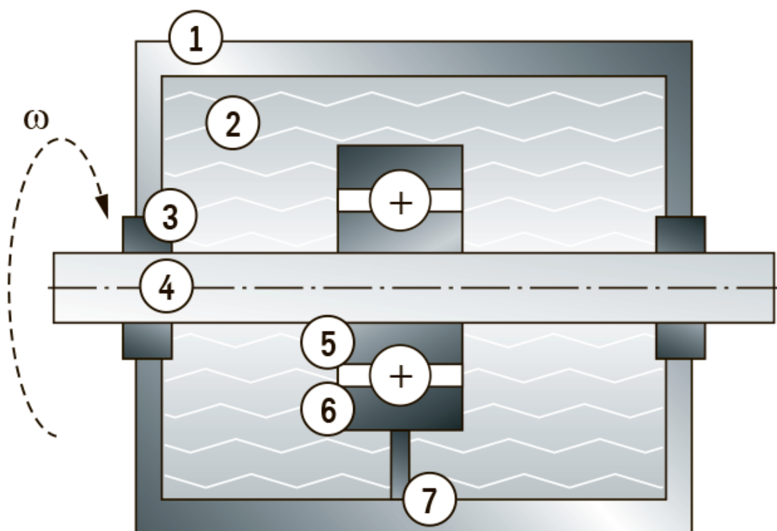
Рис. 19. Модель устройства для испытания подшипника в агрессивной среде с вращением подшипника через вал:
