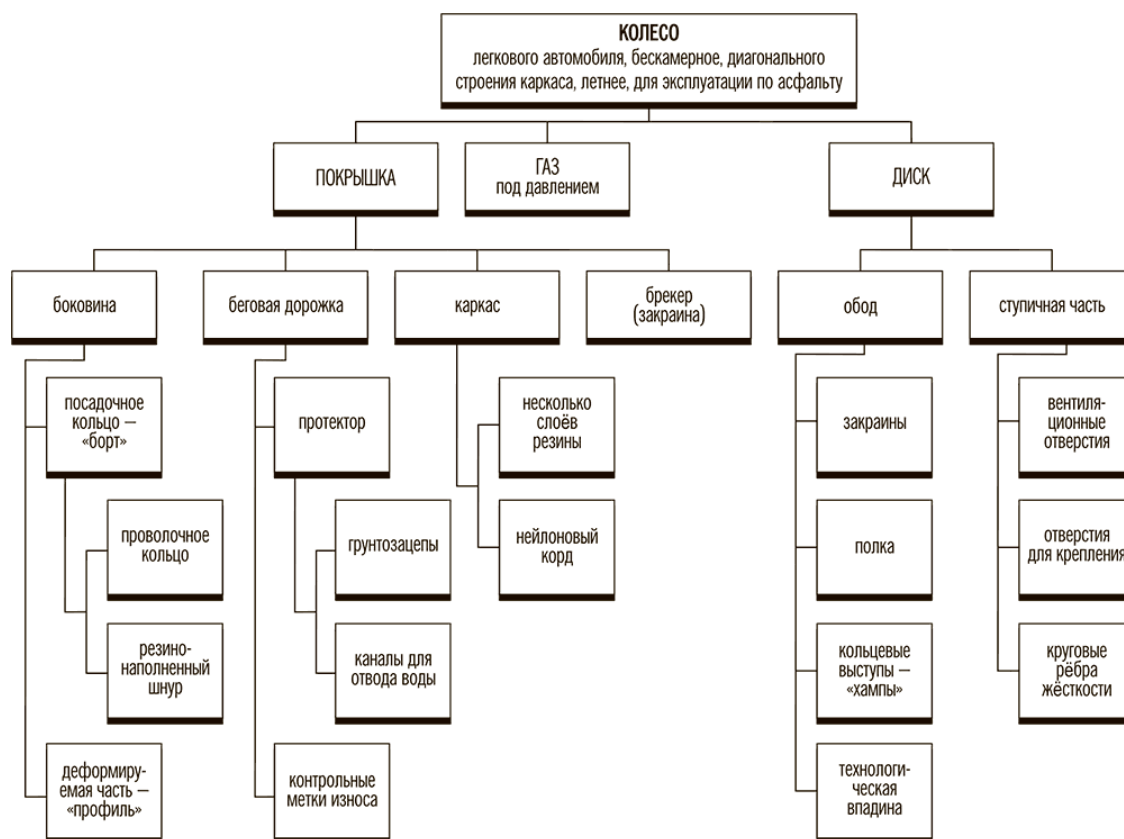
Рис. 7. Структурная схема колеса
